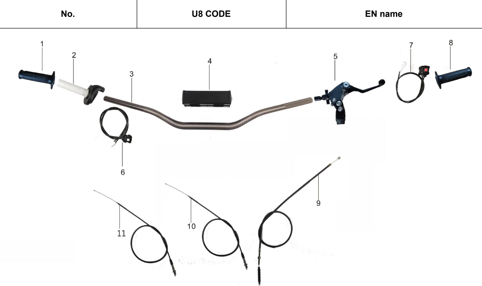
方向把总成
