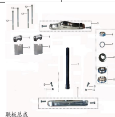
联板总成
