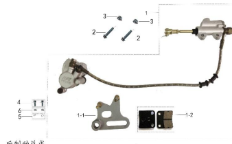
后制动总成
