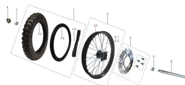
前轮总成
