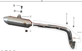
消音器总成
