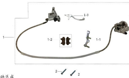
前制动总成
