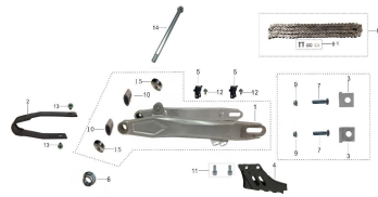
平叉总成
