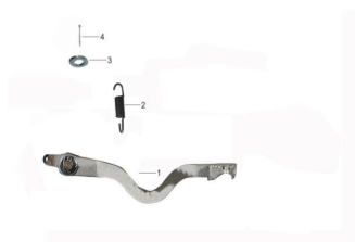
刹车踏板总成
