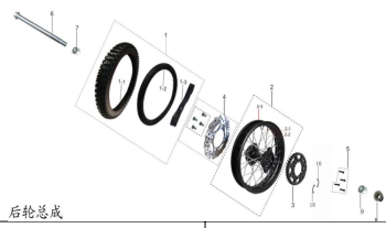
后轮总成
